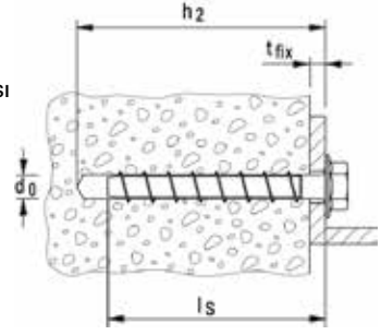
ULTRACUT FBS II US TX - Altıgen başlı beton vidası
