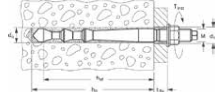
Highbond dübel FHB II-A L (uzun versiyon)
